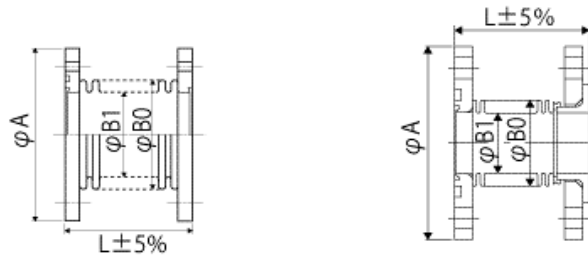
図 (左) 両端固定フランジ (右) 片側固定・片側回転フランジ
